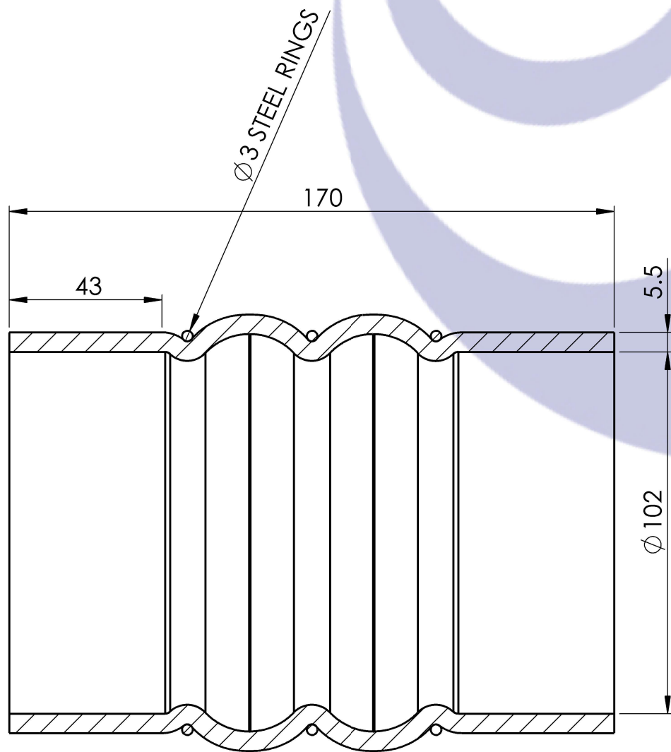
SECTION A-A
