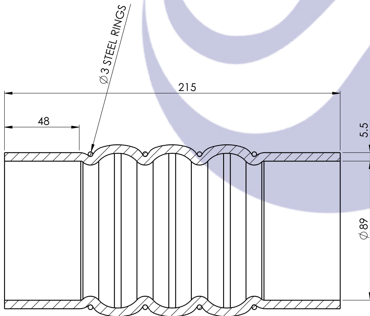
SECTION A-A
